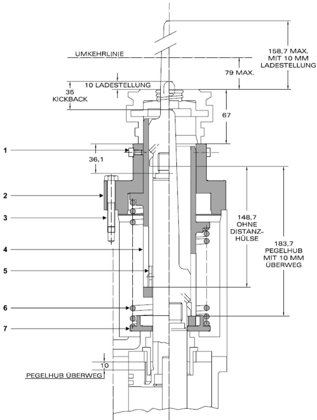
Bild 1: EPB Pegelhülse 62-404 Gr.9
